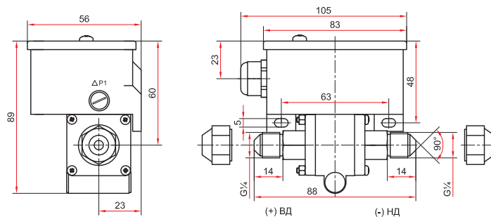
РДД-2Р с наружной резьбой с накидной гайкой G1/4
