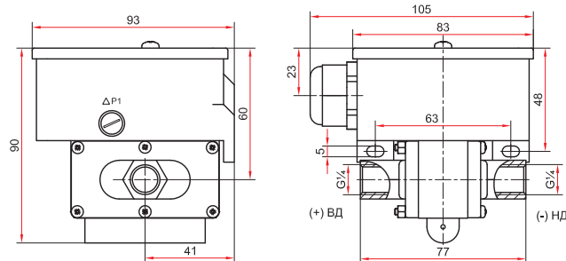
РДД-2Р с внутренней резьбой G1/4
